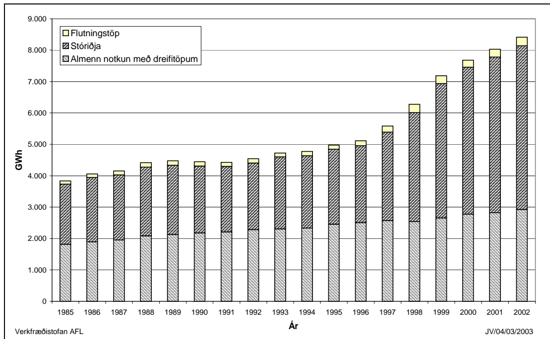
Raforkunotkun á Íslandi árin 1985-2002.
