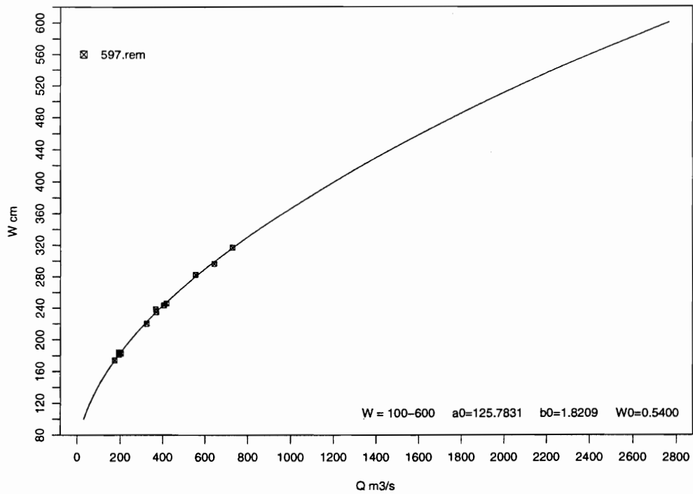
Mynd 1: Rennslislykill nr. 3 fyrir vhm 597 í Þjórsá við Tröllkonuhlaup, allt sviðið.
