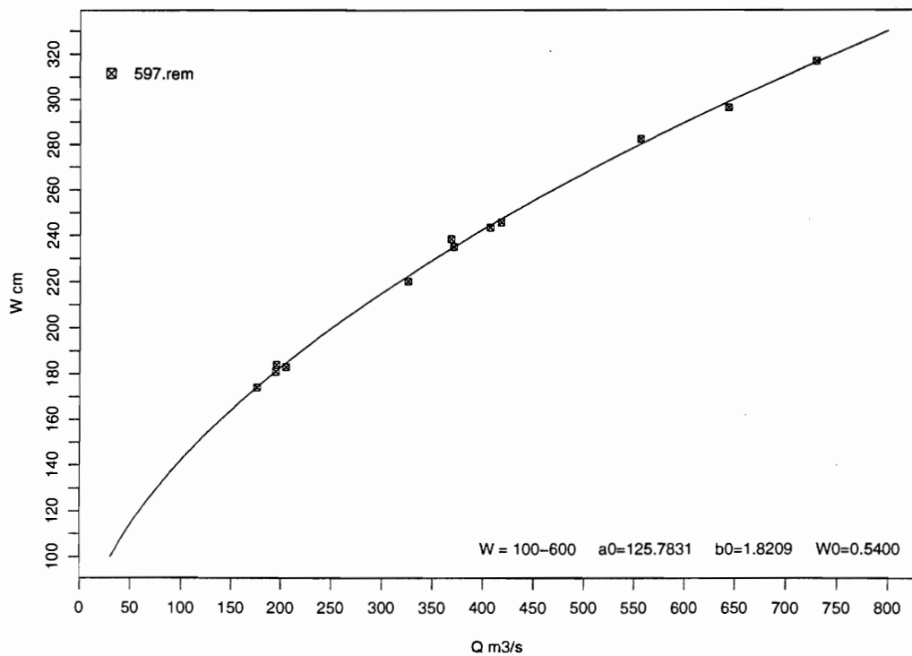
Mynd 2: Rennslislykill nr. 3 fyrir vhm 597 í Þjórsá við Tröllkonuhlaup, mælt svið.
