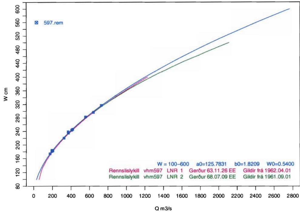
Mynd 3: Samanburður rennslislykla fyrir vhm 597 í Þjórsá við Tröllkonuhlaup, allt sviðið.
