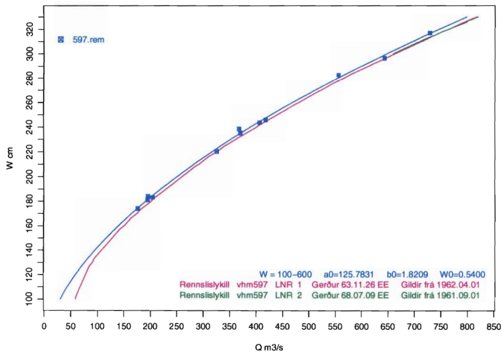
Mynd 4: Samanburður rennslislykla fyrir vhm 597 í Þjórsá við Tröllkonuhlaup, mælt sviði.
