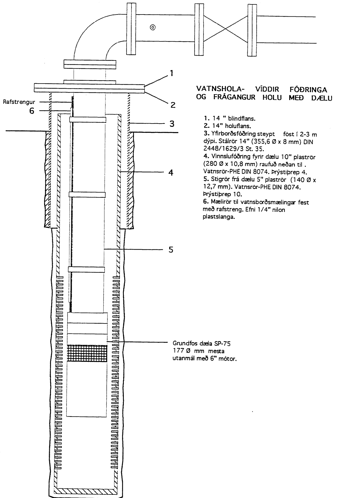
Mynd 5. Víddir fóðringa og frágangur holu með dælu.
