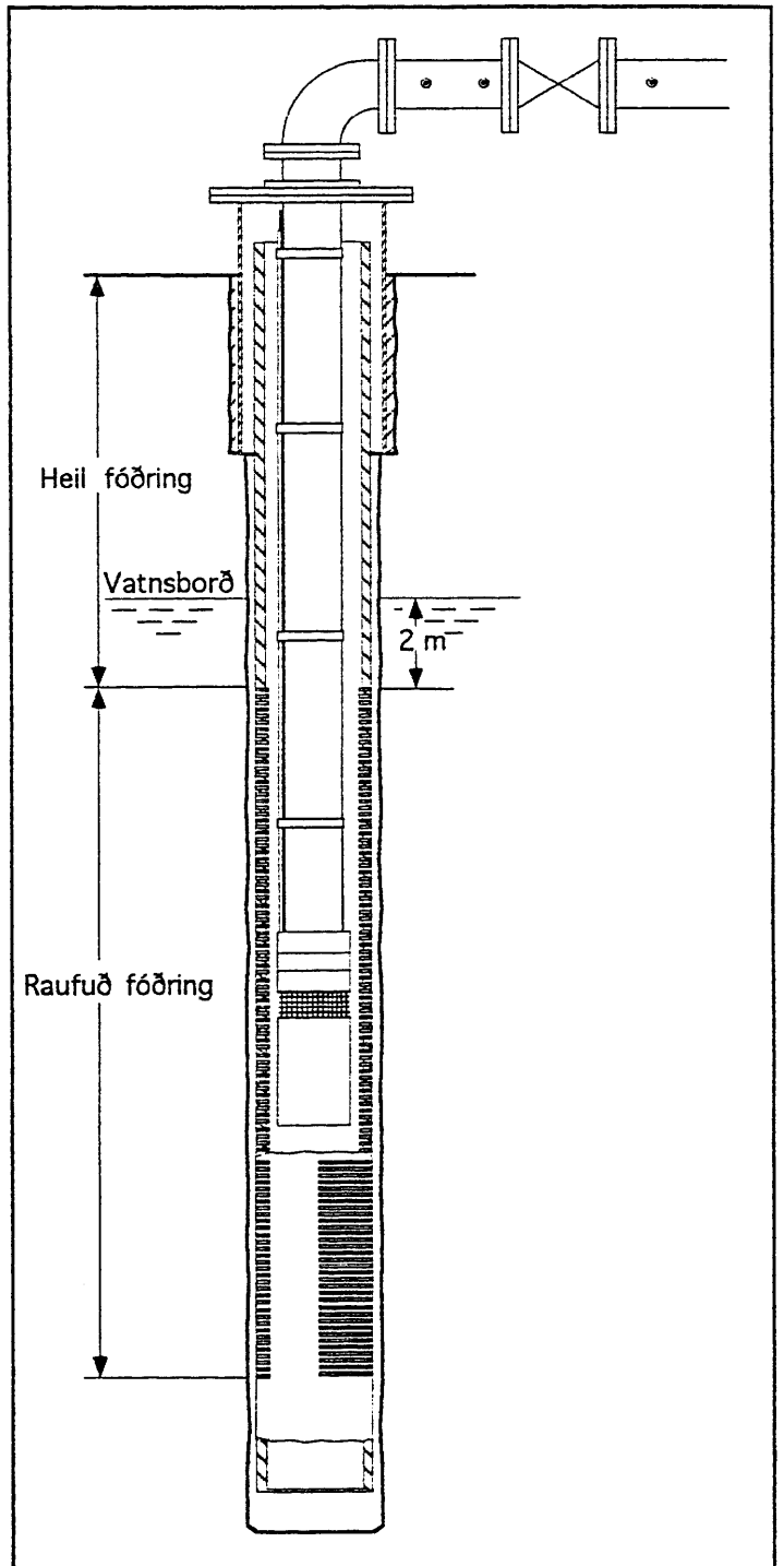
Mynd 3. Lokafrágangur holunnar
