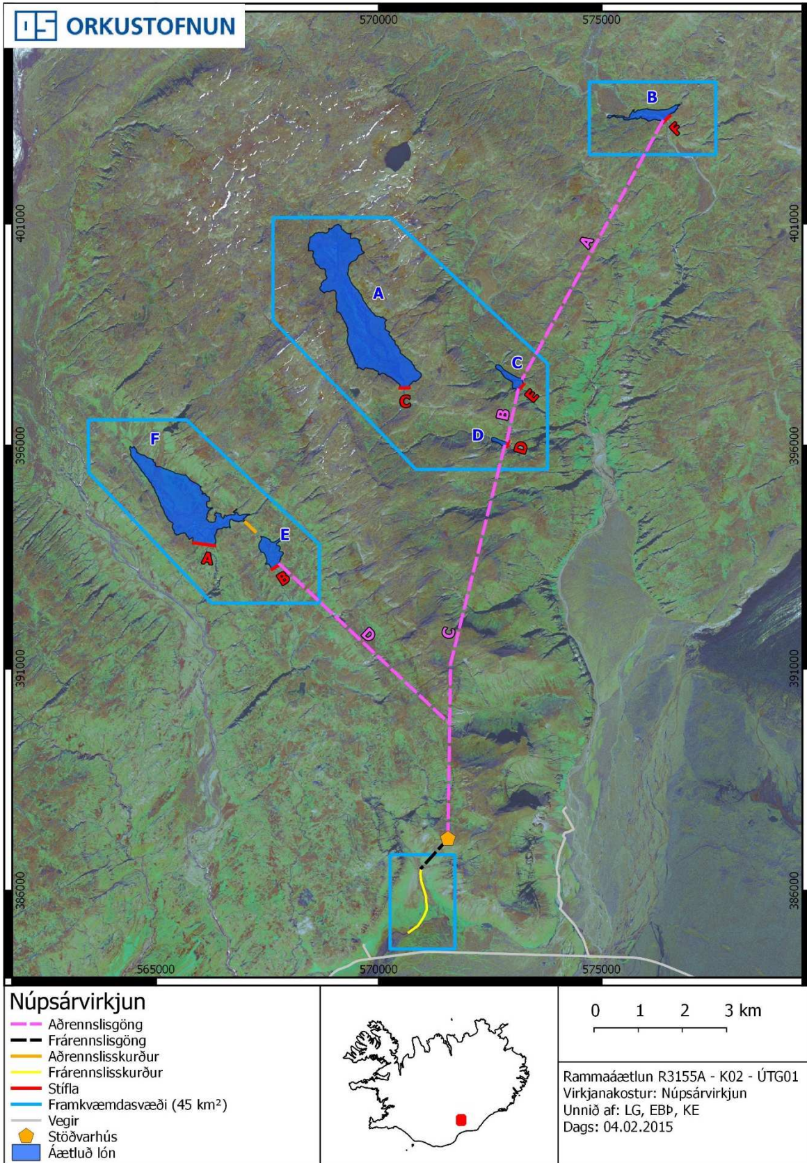
Mynd 6.53-3 Loftmynd af Núpsárvirksjun og helstu mannvirkjum tengdum virksjuninni
