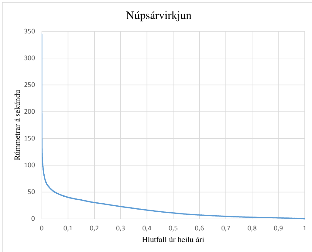
Mynd 6.53-1 Langæislína fyrir Núpsárvirkjun
