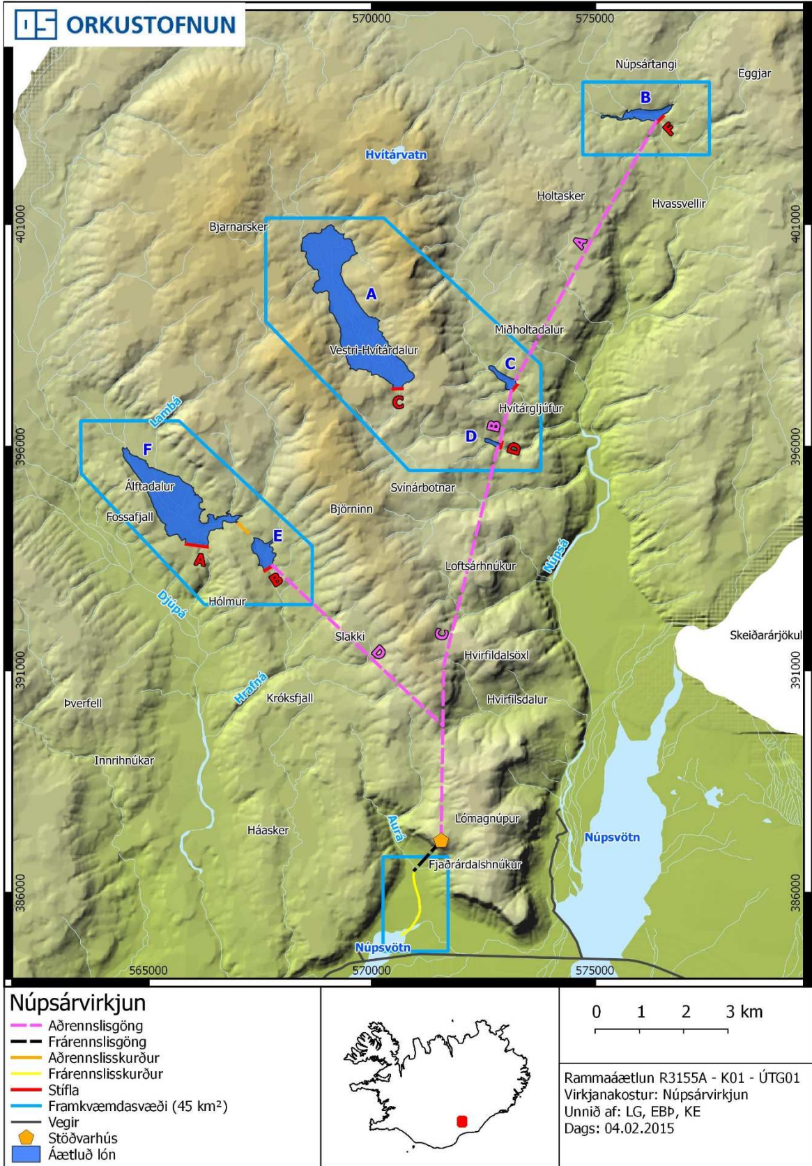
Mynd 6.53-2 Kort af Núpsárvirkjun og helstu mannvirkjum tengdum virkjuninni
