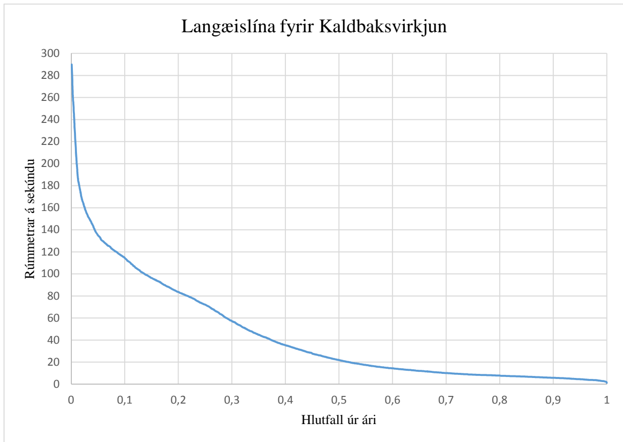
Mynd 6.49-1 Langæislína fyrir Kaldbaksvirkjun
