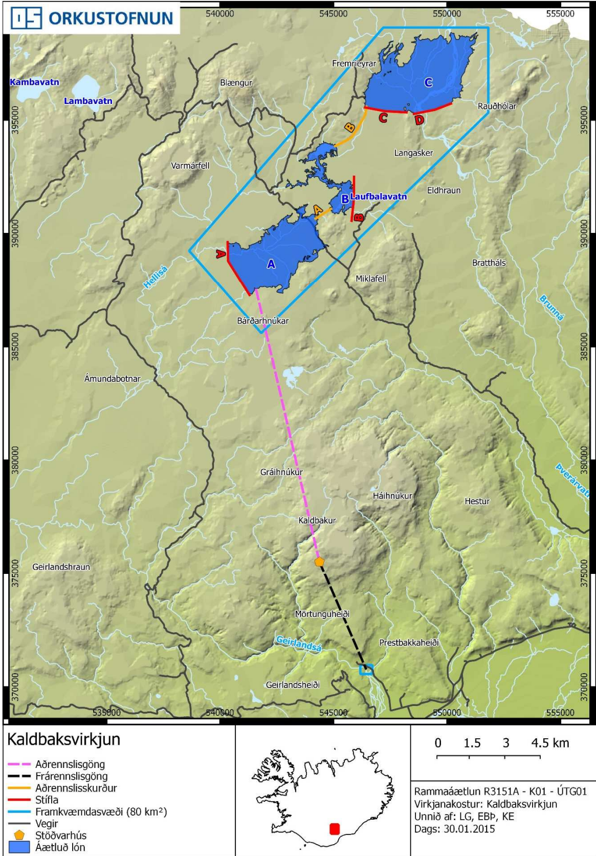
Mynd 6.49-2 Kort af Kaldbaksvirkjun og helstu mannvirkjum tengdum virkjuninni
