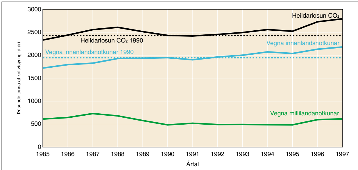
Mynd 3.4 Losun koltvísyrings frá brennslu eldsneytis 1985–1997.
