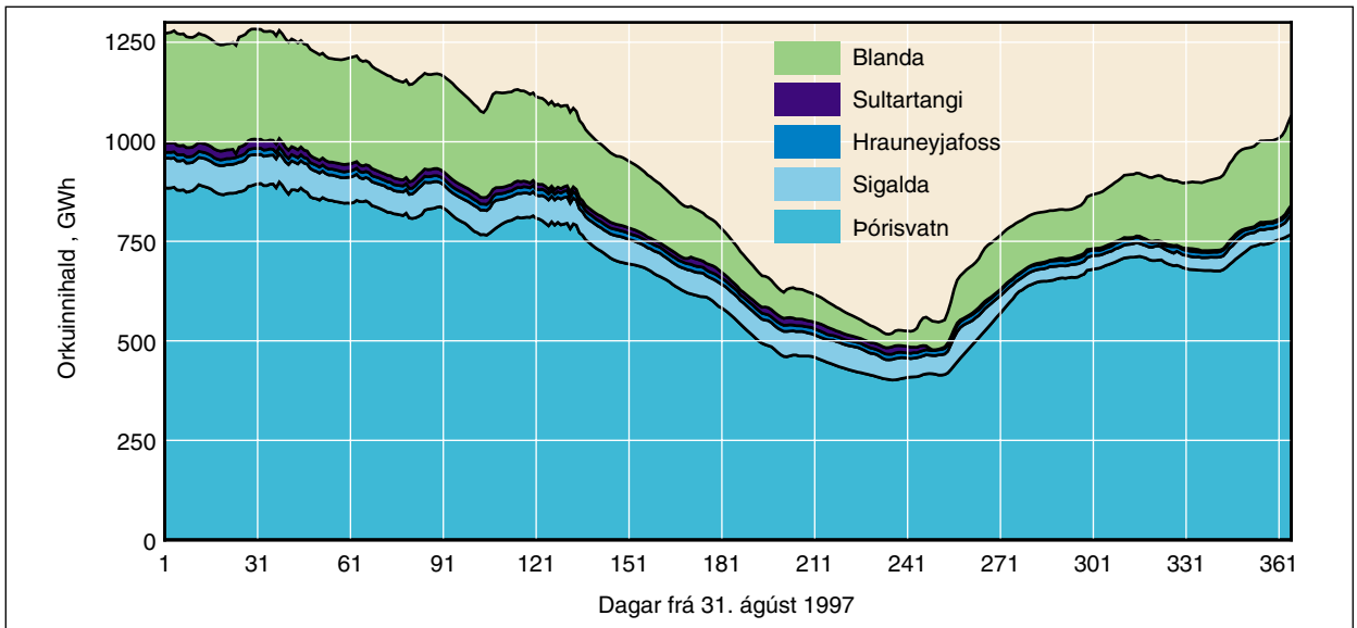
Mynd 1.6 Rekstur miðlunarlóna 1997–1998.
